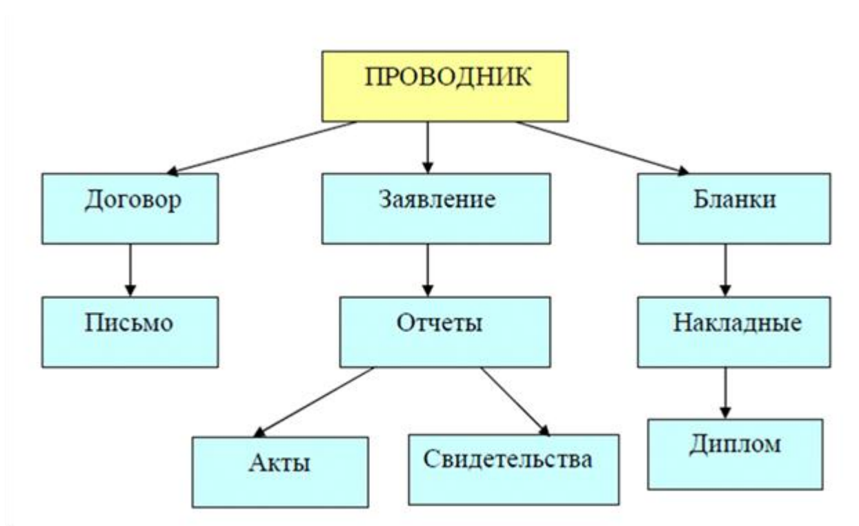
Рис. 1. Структура каталогов
